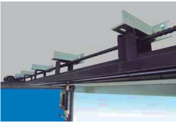
Detalle de la guía superior específicamente fabricado para cada puerta en particular.
