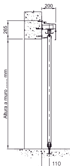
Corredera de dos hojas con guía sobre pavimento.
