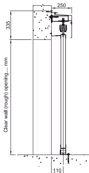
SECCION VERTICAL CORREDERA SOBRE PAVIMENTO
