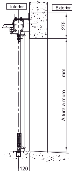
SECCION VERTICAL ANCLAJE ESTANDAR
