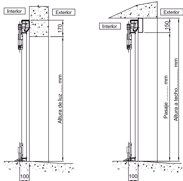
SECCION VERTICAL ANCLAJE ESTANDAR
