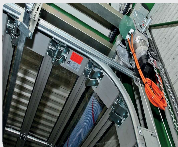
Moteur de porte sectionnelle à grande vitesse
