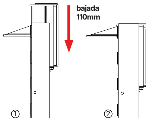
Accionamiento mecánico de bajada del tope de muelle de carga
